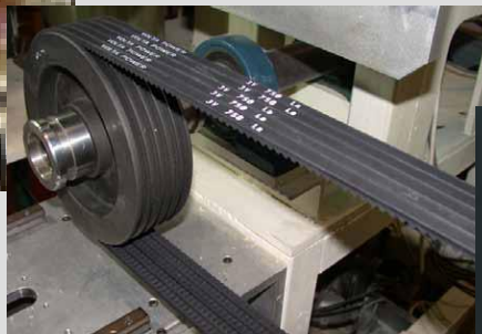
Ιμάντες ισχύος
